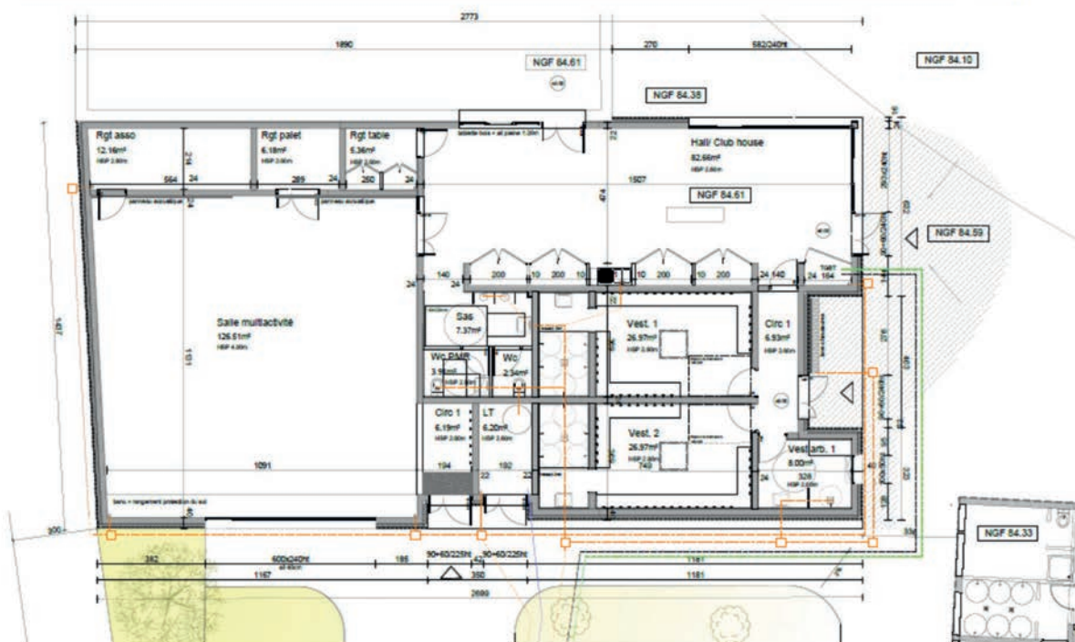
PLAN REZ-DE-CHAUSSEE 1-100°
